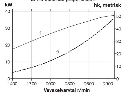
Effekt 1. Vevaxeleffekt 2. Vid beräknad propellerlast x^{2.5}
