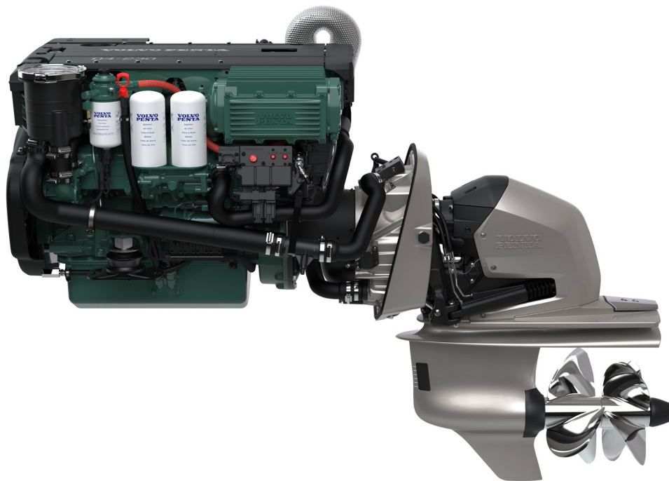
Effekt Vevaxe effekt Vid beräknad propellerlast x 2,5
