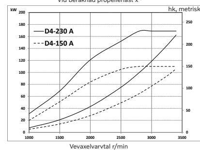
Vridmoment Vridmoment mätt på vevaxeln
